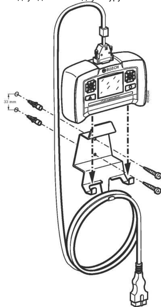
Рис. 2. Монтаж узла крепления к стене.
