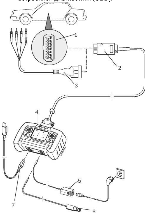
Рис. 3. Схема подключения KTS 200:
